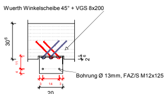
BEISPIEL EINES EINZELELEMENTPLANS, WELCHER ZUR ARBEITSVORBEREITUNG IN DIE PRODUKTION WEITERGEGEBEN WIRD.
