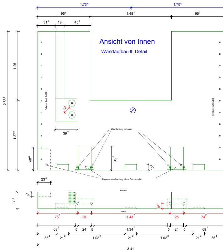
BEISPIEL EINES EINZELELEMENTPLANS, WELCHER ZUR ARBEITSVORBEREITUNG IN DIE PRODUKTION WEITERGEGEBEN WIRD.
