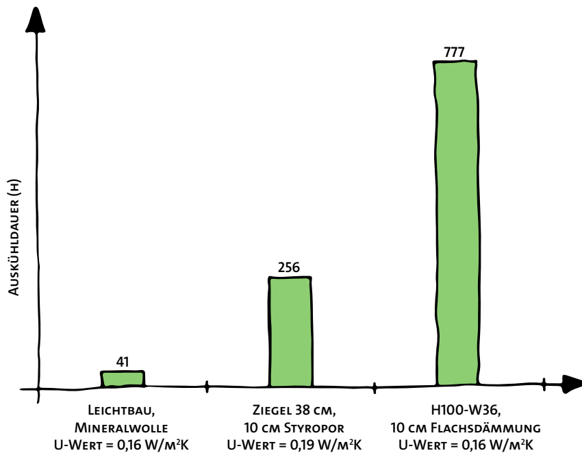
VERGLEICH DER AUSKÜHLZEIT 3ER KONSTRUKTIONEN MIT EINEM ÄHNLICHEN U-WERT (TU GRAZ, THERMISCHE SIMULATION ZUM HOLZ100 BAUSYSTEM, 2001)
